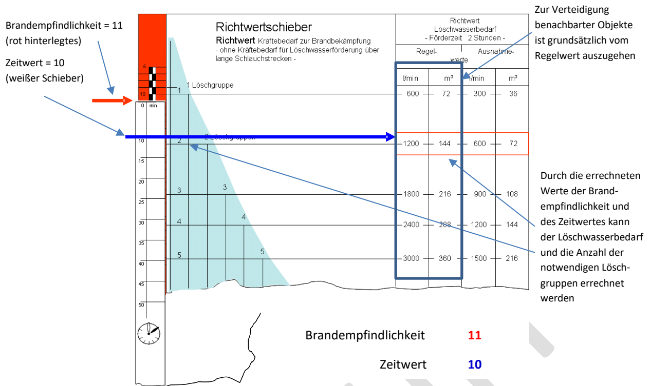
Abbildung 35 Richtwertverfahren erforderliches Löschwasser und Löschgruppen
