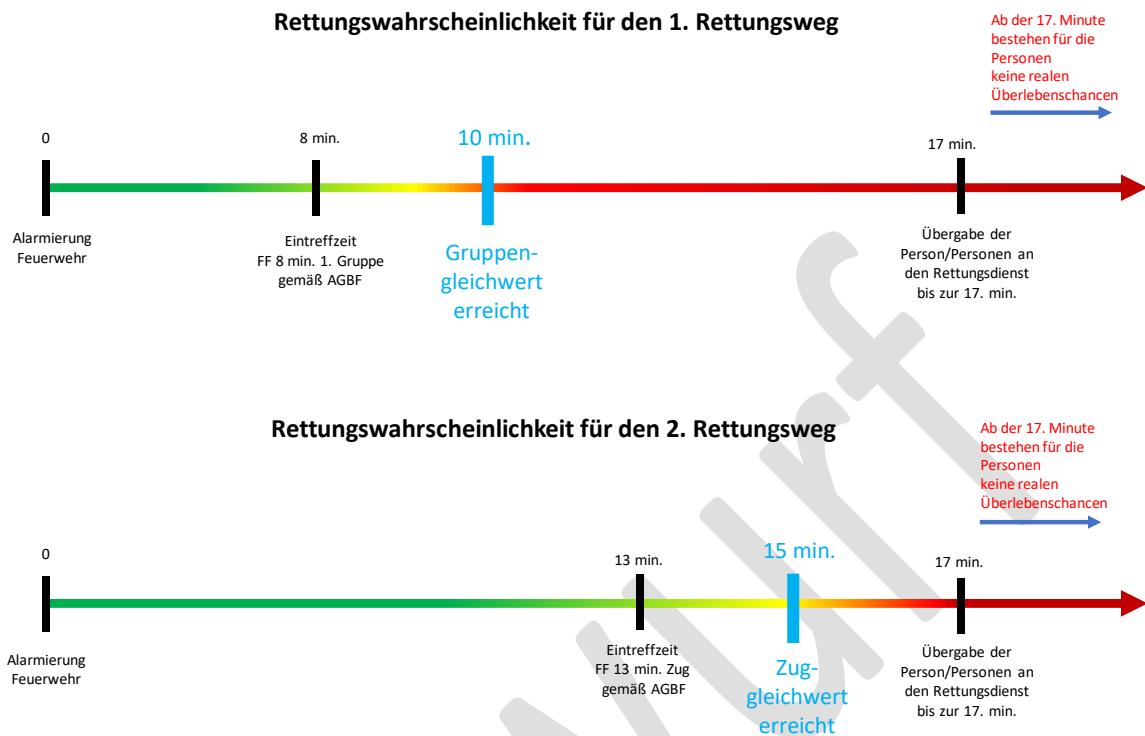
Abbildung 27 Muster 1. und 2. Rettungsweg
