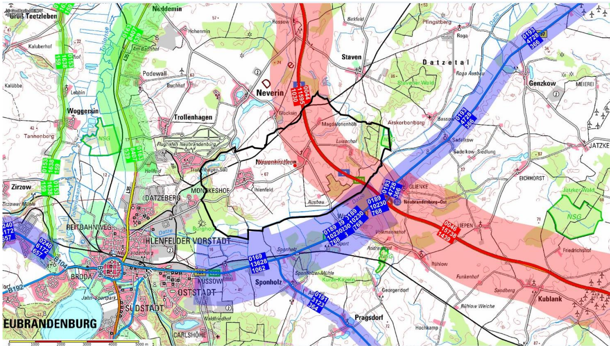
Abbildung 4 Verkehrsführung Gemeinde Neuenkirchen [6]
